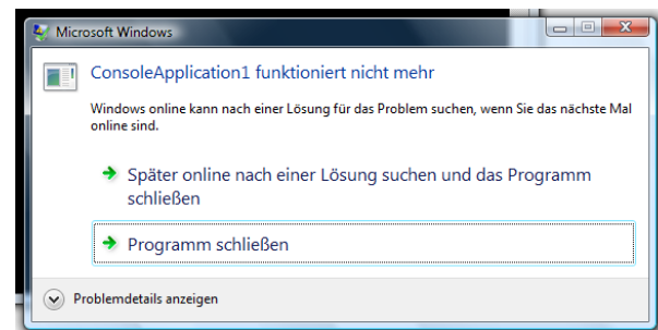
Abbildung 6 Abgestürzte Konsolenanwendung
